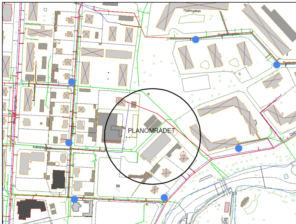
Befintliga VA-ledningar (vatten=blå, dagvatten=gröna, spillvatten=röda) samt brandposter (blå cirklar) i planområdets närhet.
