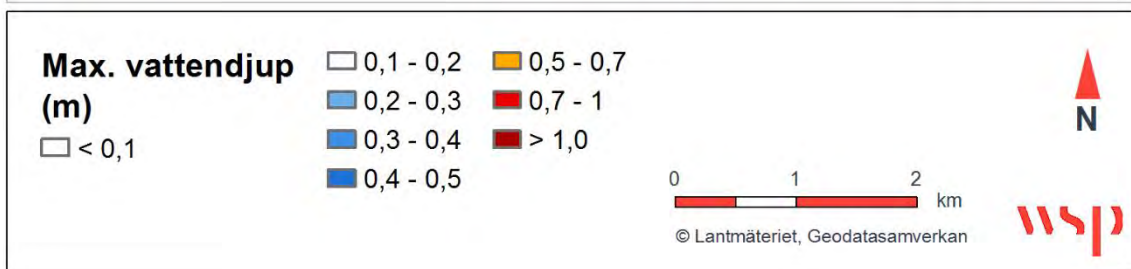
Figur 20: Beräknade maximalt vattendjup vid ett klimatanpassat 100-årsregn, Område 8.
