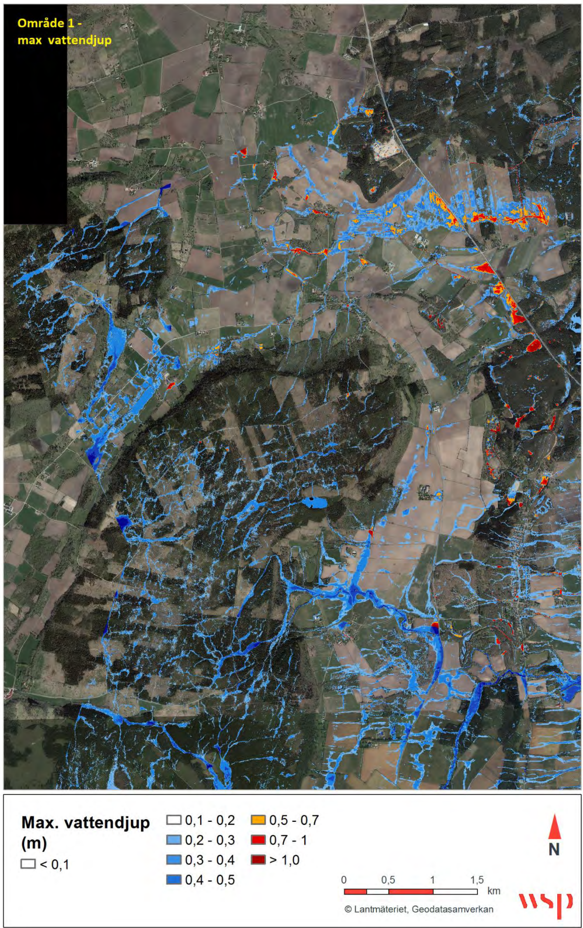
Figur 6: Beräknade maximalt vattendjup vid ett klimatanpassat 100-årsregn. Område 1.
