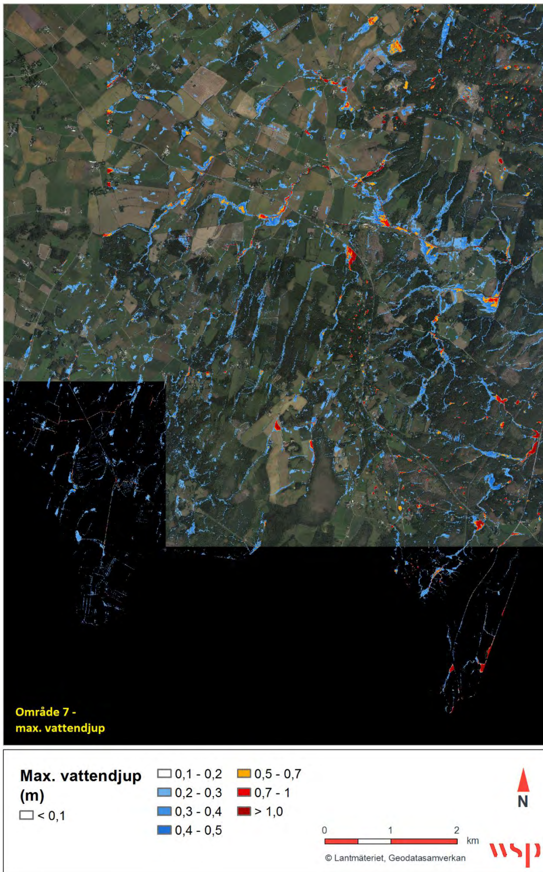
Figur 18: Beräknade maximalt vattendjup vid ett klimatanpassat 100-årsregn, Område 7.
