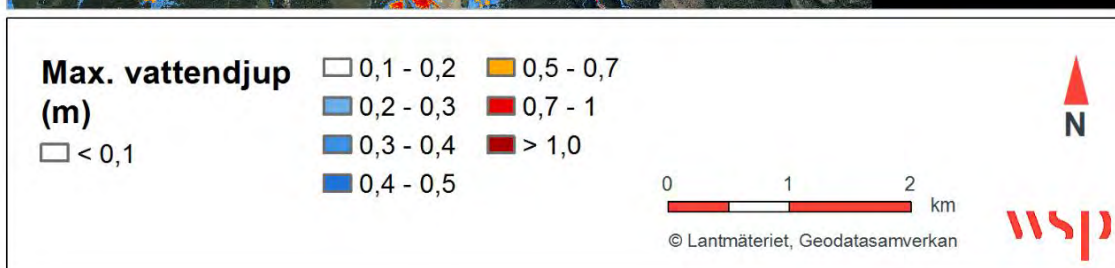
Figur 10: Beräknade maximalt vattendjup vid ett klimatanpassat 100-årsregn, Område 3.
